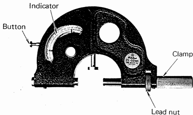
Fig. 7 Snap meter
